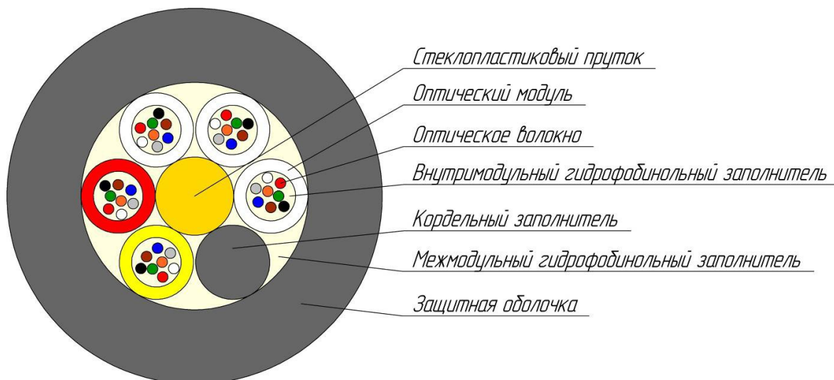
Кабель ОКГнг(А)-HF-0,22-2...48П
